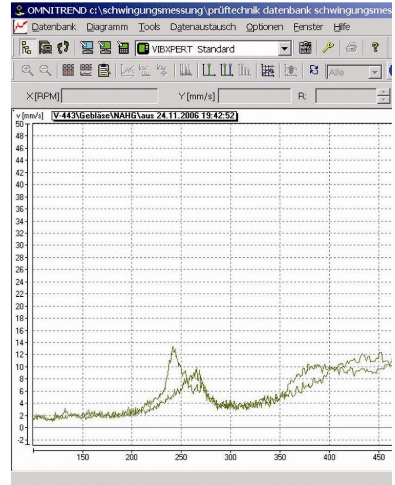
Messergebnis einer Auslaufkurvenanalyse
